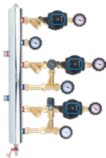
BPS на 3 контура с насосами AFRISO APH
