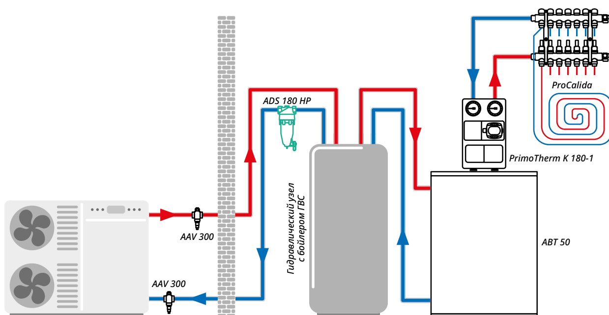
Универсальный сепаратор шлама ADS 180 HP, используемый в системе с моноблочным тепловым насосом
