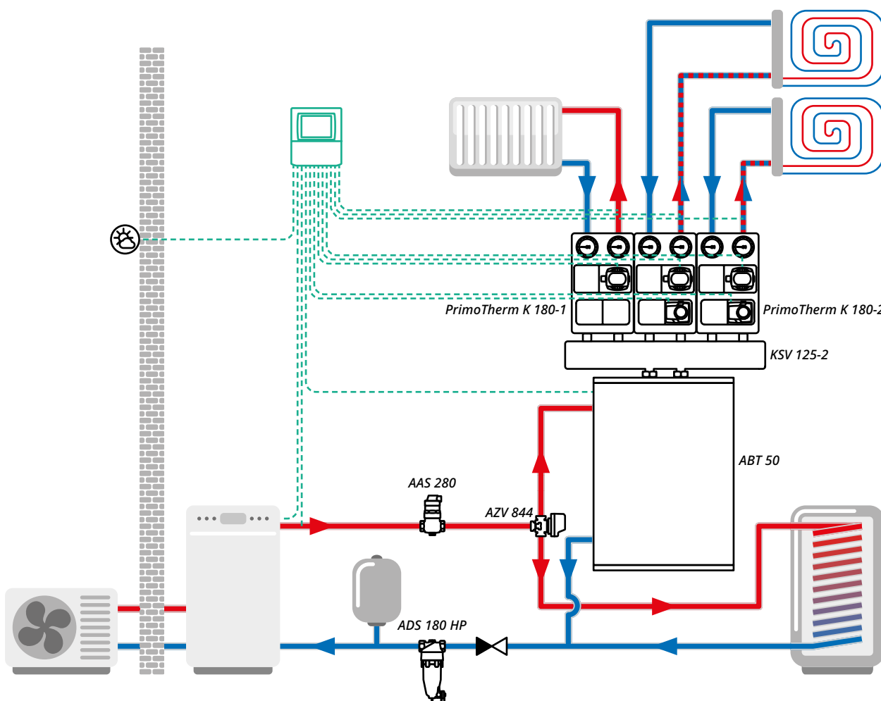
Контроллер BWC 330 Pro, установленный в системе с тепловым насосом и тремя контурами: одним радиаторным и двумя контурами теплого пола. В системе с таким источником тепла контроллер не управляет наполнением бойлера ГВС – каждый тепловой насос имеет эту функцию встроенной.
