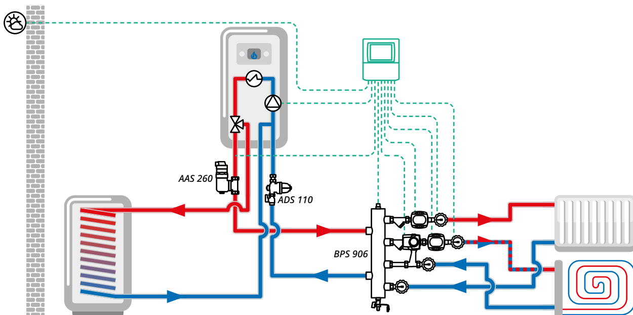
Контроллер BWC 330 Pro, установленный в системе с газовым/электрическим котлом и двумя контурами: радиаторным и теплым полом. В системе с таким источником тепла контроллер не управляет наполнением бойлера ГВС – каждый котел имеет эту функцию встроенной.
