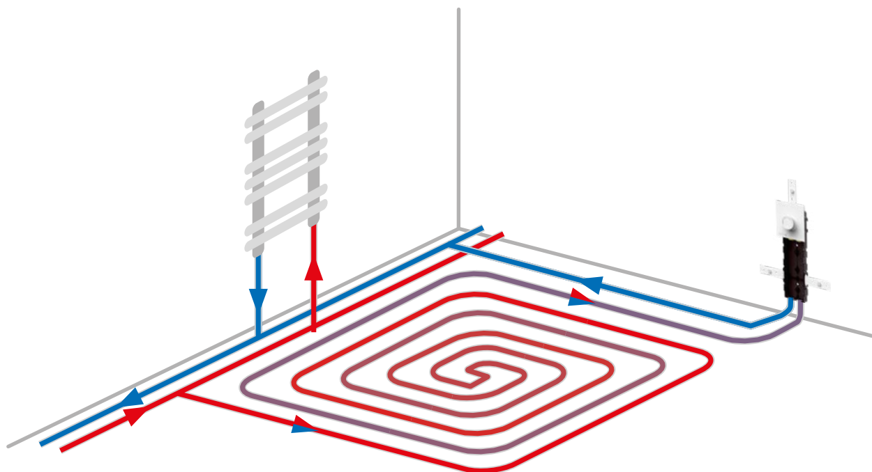
Схема применения
