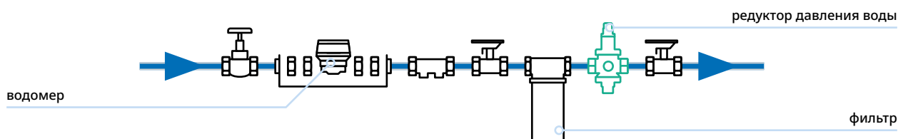
Подключение к водопроводу в частном доме
