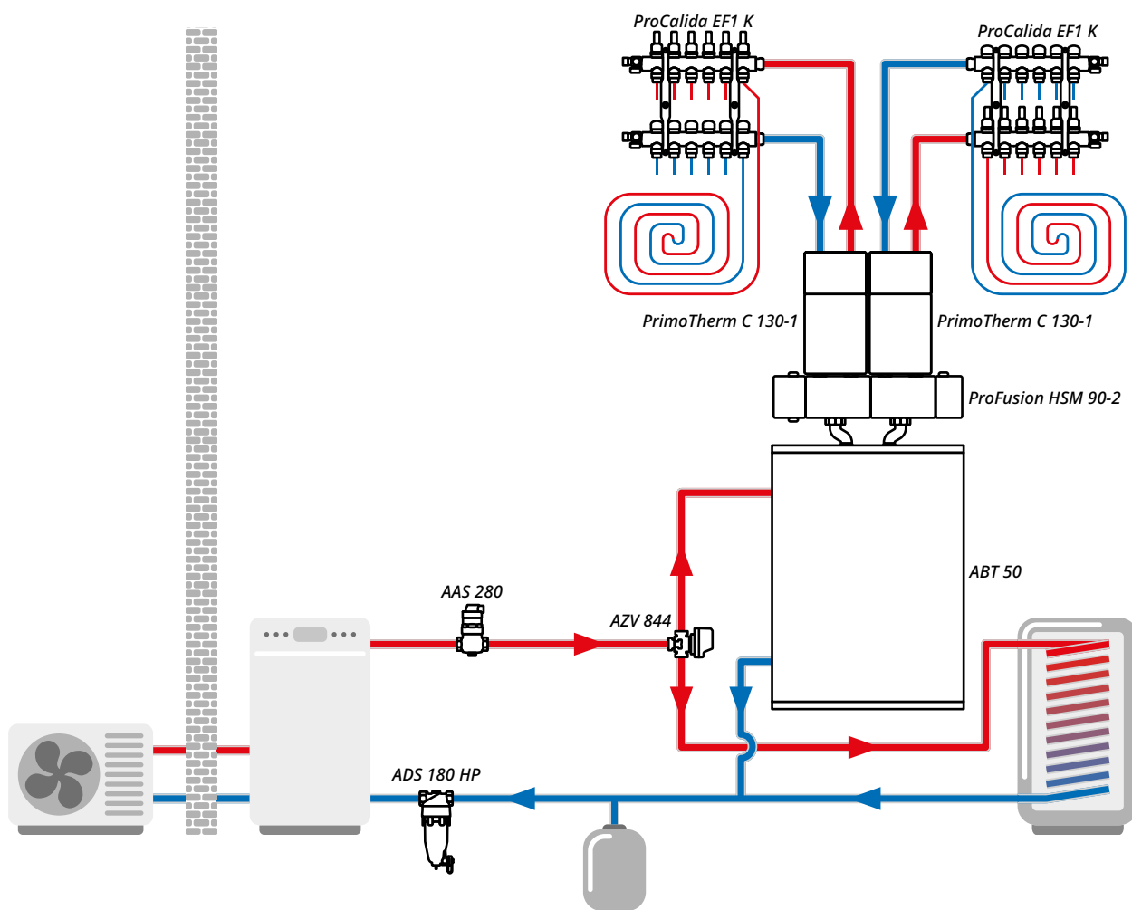
Схема использования двух насосных групп PrimoTherm C с подмесом, установленных на коллекторе ProFusion HSM 90. Коллектор с помощью эксцентриков закреплен на буферной емкости
