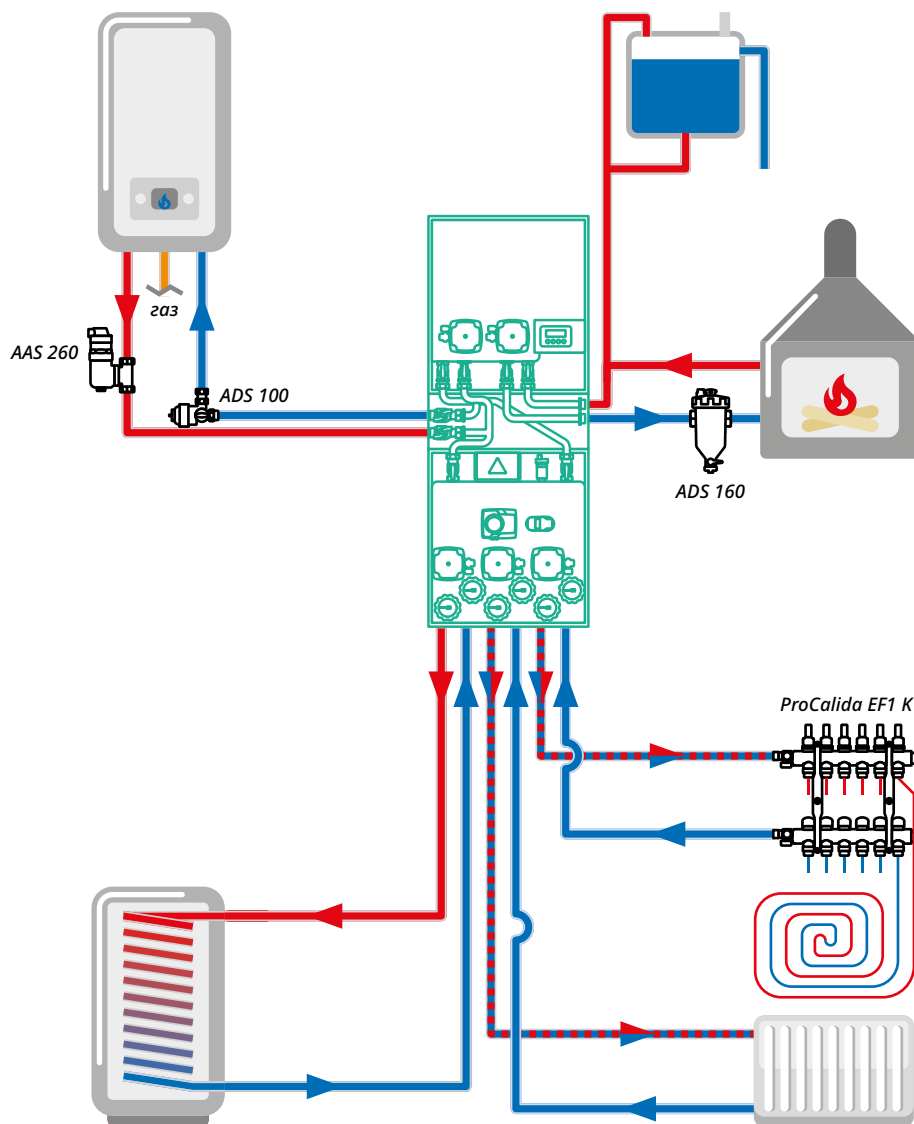
Схема использования комплекта наборов PrimoBox AHB 622 + AJB + AZB 351
