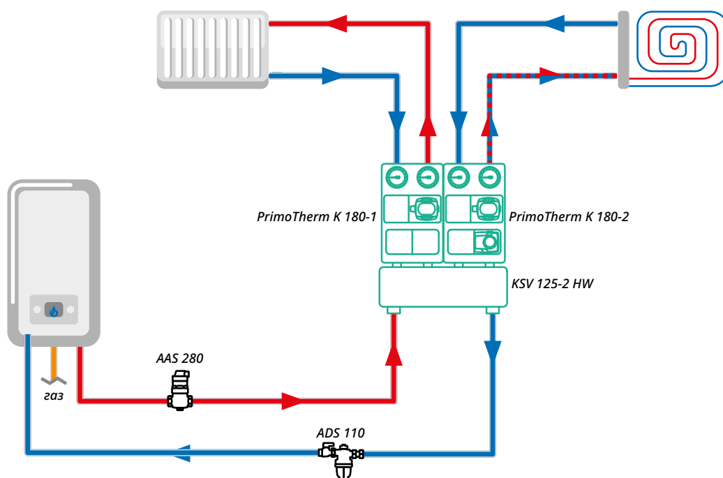
Схема использования двух насосных групп PrimoTherm, прямой и с подмесом, установленных на коллекторе KSV
