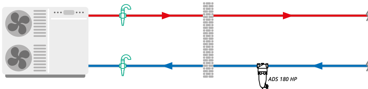
Пример схемы применения клапанов AAV
