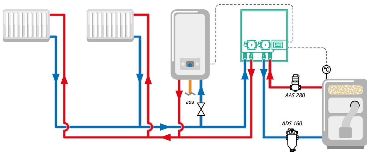
Схема использования разделительного набора PrimoBox AHB 622
