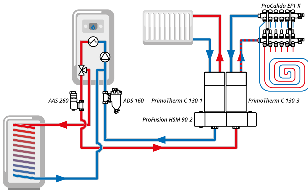
Схема использования двух насосных групп PrimoTherm C, прямой и с подмесом, установленных на коллекторе ProFusion HSM 90
