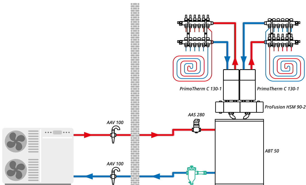
Комплект сервисной арматуры для тепловых насосов AHS в системе с моноблочным тепловым насосом
