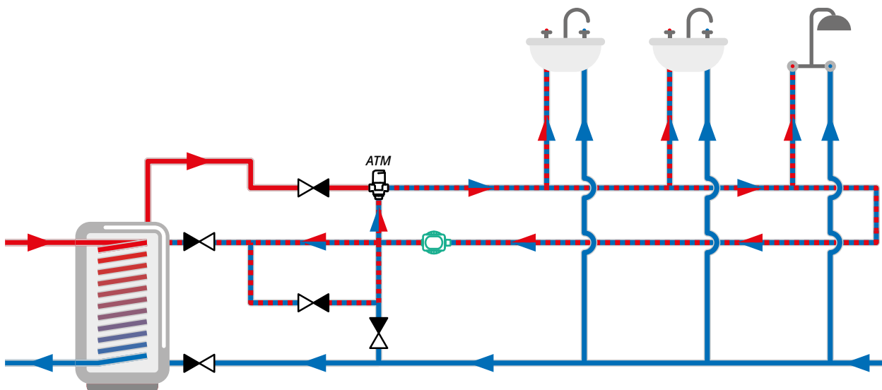
Насос APW 710, установленный в системе циркуляции ГВС с термостатическим клапаном ATM
