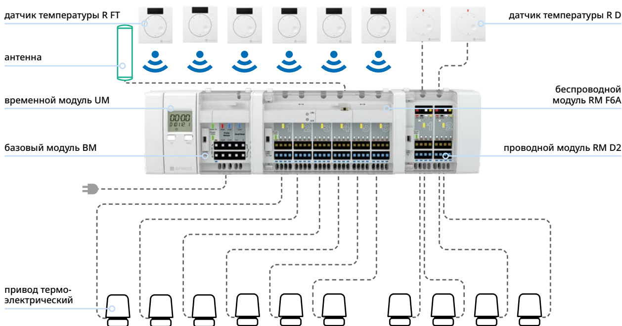
Пример схемы применения системы управления поверхностным отоплением и охлаждением CosiTherm
