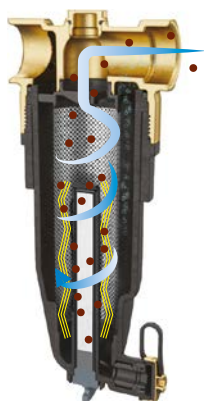
Шаг 1: притяжение загрязнений магнитом.
