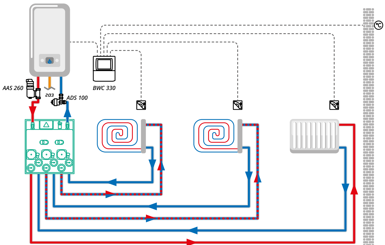
Схема использования смесительного набора на три контура PrimoBox AZB 311
