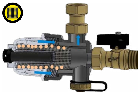
Шаг 2: отложение загрязнений на сетке фильтра.
