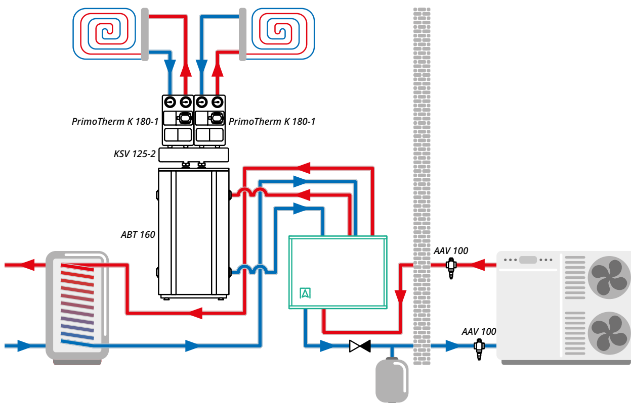
Гидравлический набор AMB 900, используемый в системе с моноблочным тепловым насосом и двумя контурами поверхностного отопления
