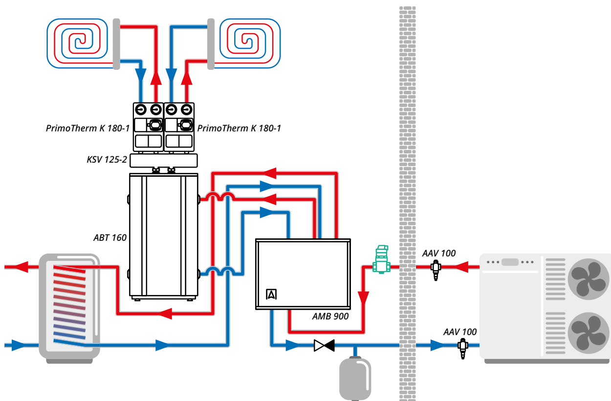
Сепаратор воздуха, используемый в системе с тепловым насосом моноблочного типа
