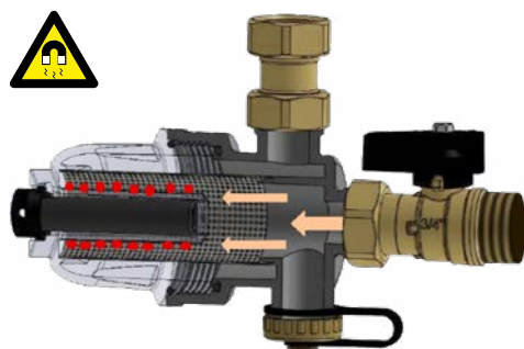
Шаг 1: магнит притягивает загрязнения.
