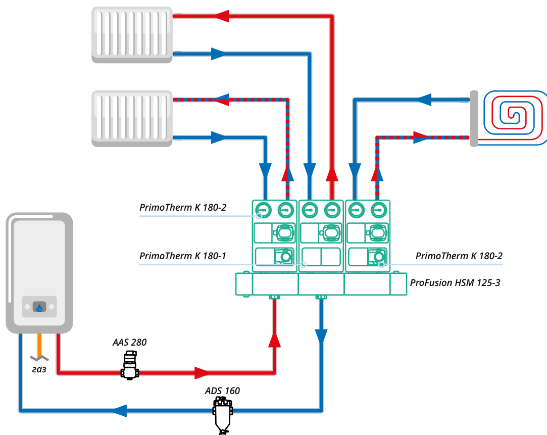
Схема использования трех насосных групп PrimoTherm, прямой и двух с подмесом, установленных на коллекторе ProFusion HSM 125
