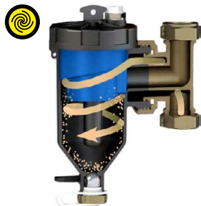
Шаг 1: введение теплоносителя в вихревое движение.
