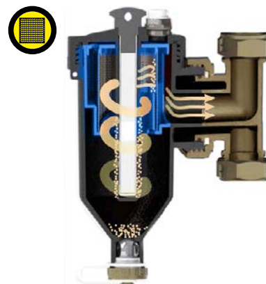
Шаг 3: отложение загрязнений на сетке фильтра.
