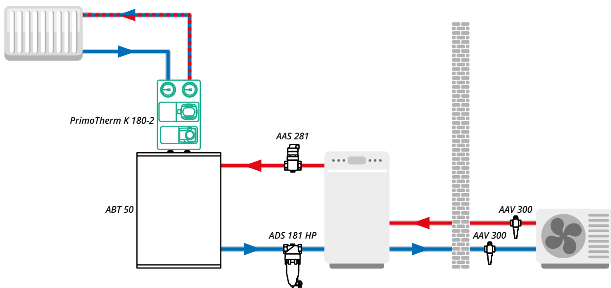
Схема использования отдельной группы PrimoTherm с подмесом, установленной на буферной емкости
