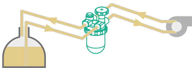
Стандартное применение двухтрубного фильтра
